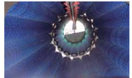
Widok wnętrza urządzenia Mega-Polisher
